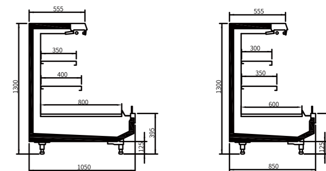
腾跃系列半高敞开式冷藏立柜
